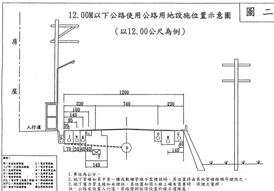
第十四條附圖二：12.00M 以下公路使用公路用地設施位置示意圖
