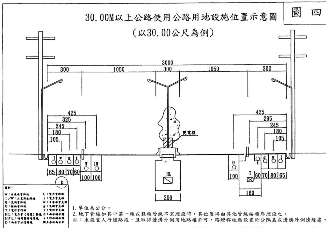
第十四條附圖四：30.00M 以上公路使用公路用地設施位置示意圖
