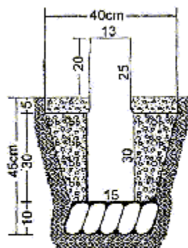
三等三角點
