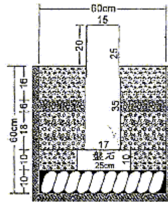
二等三角點
