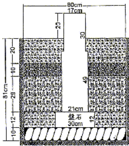
一等三角點
