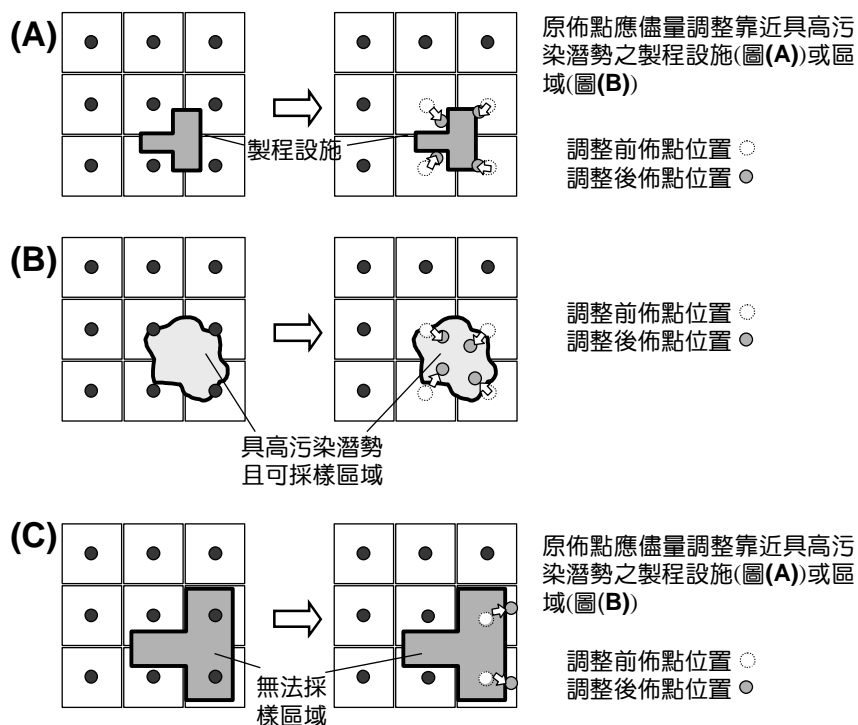
圖四、佈點位置調整示意圖
