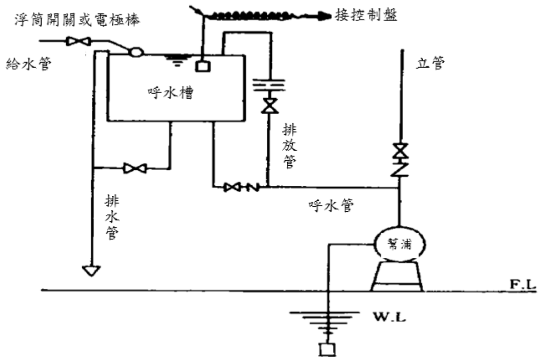
圖 2-4 呼水裝置
