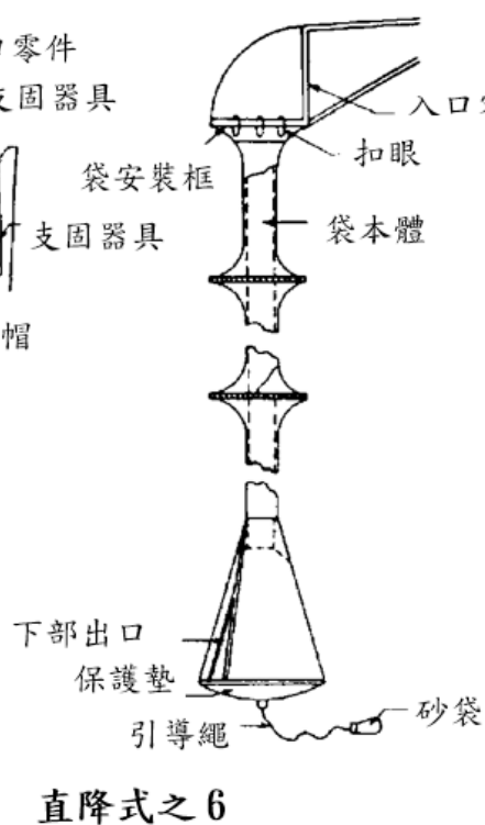
圖18-5 救助袋(例)
