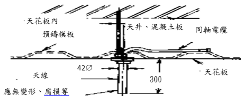
圖 24-4 天線
