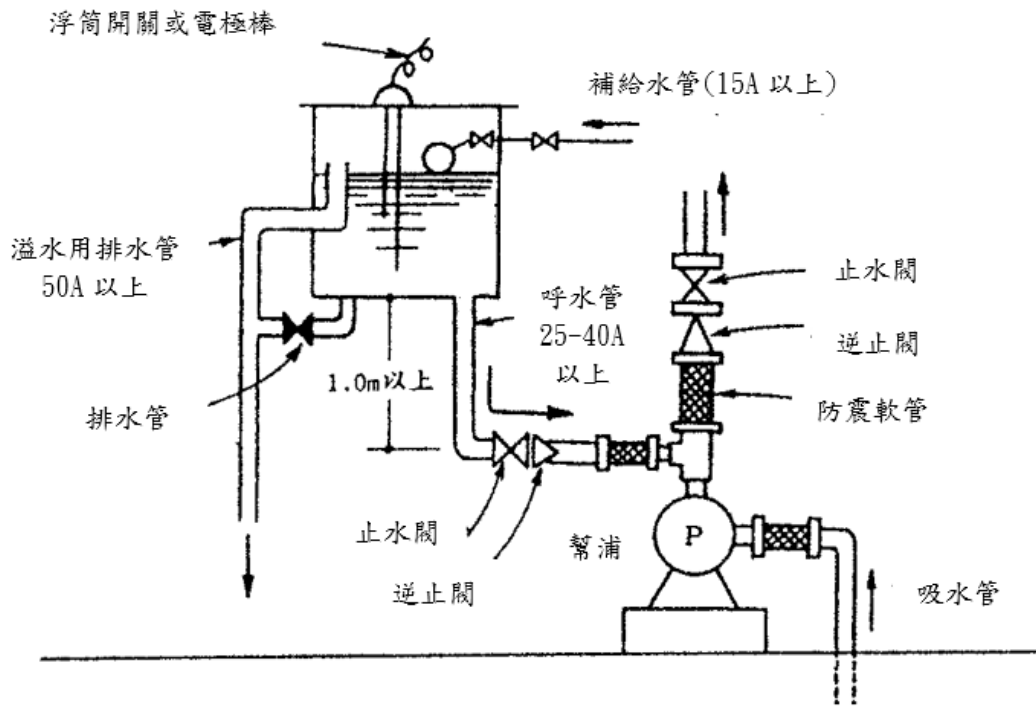
圖 21-2 呼水裝置
