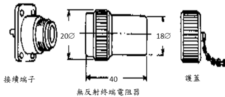
圖 24-3 端子
