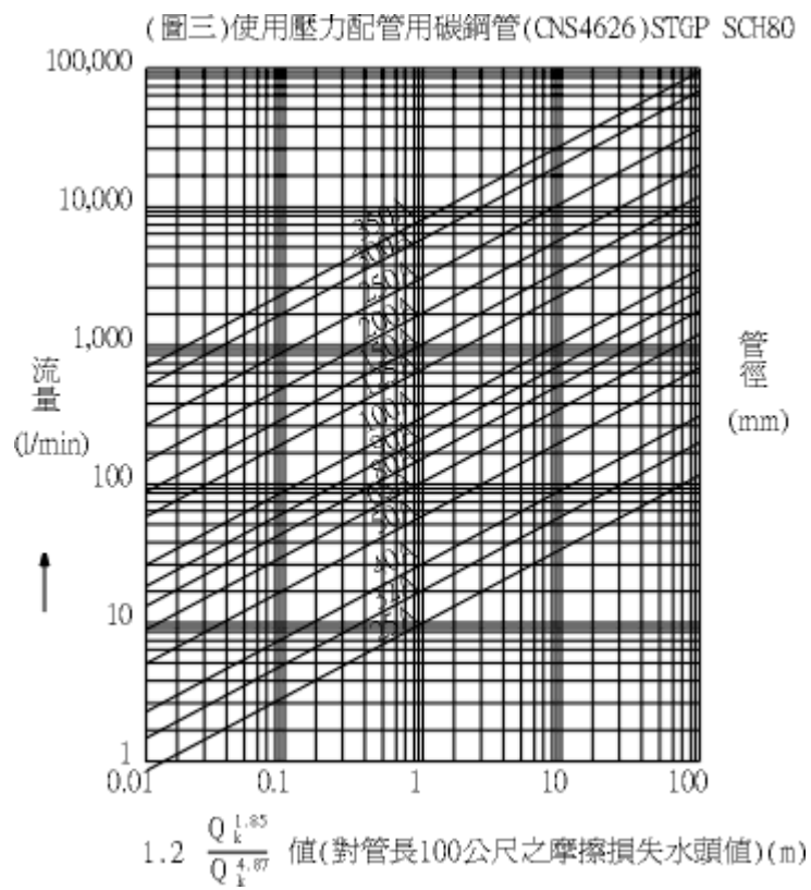
〈圖三〉使用壓力配管用碳鋼管 (CNS4626) STGPSCH80
