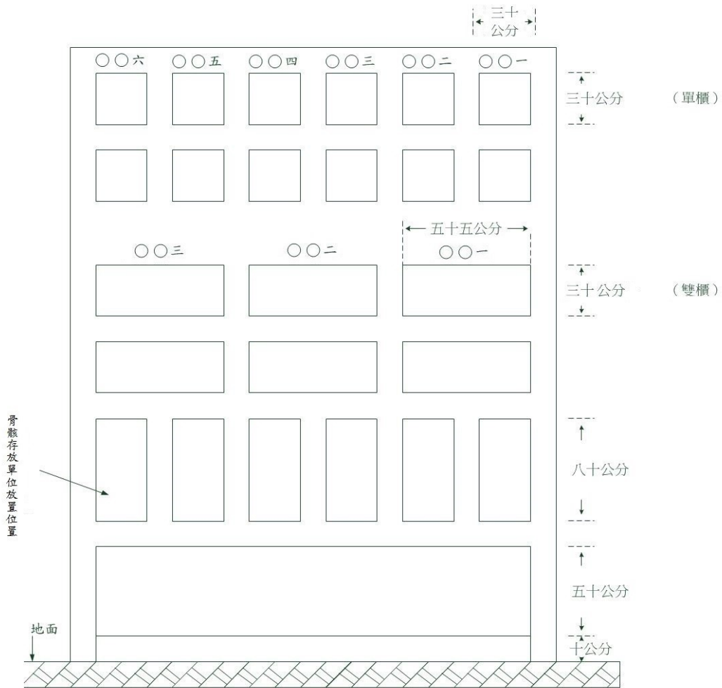
骨灰（骸）存放單位架（櫃）正面圖
